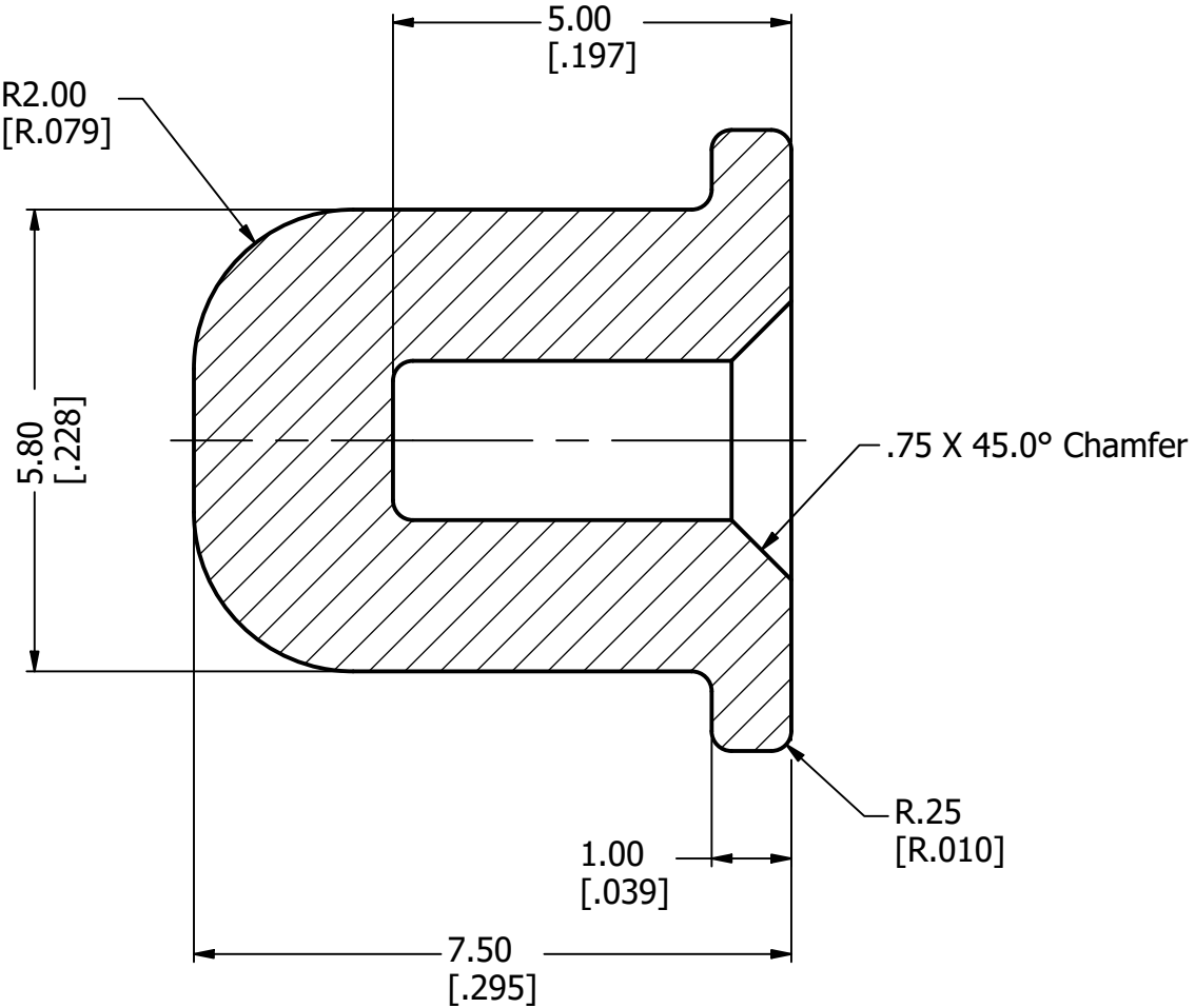
SECTION D-D SCALE 10 : 1
